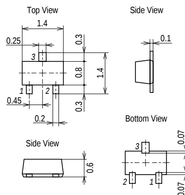
外形図 2207A (unit : mm)
