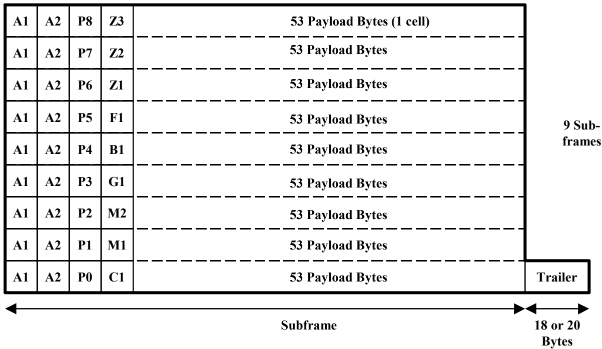
Figure 10-17. E3 PLCP Frame
