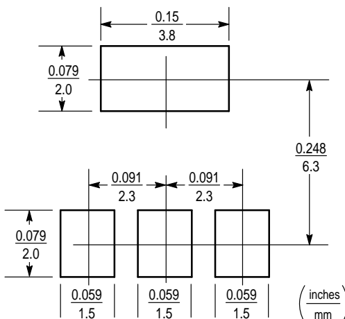
SOT-223
