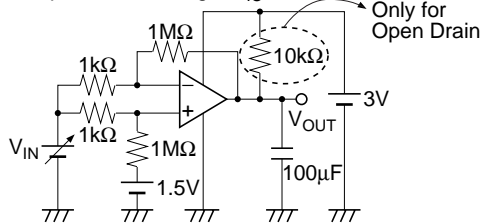
7. Input Offset Voltage, V_{IO}
