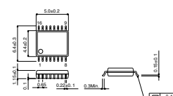
SSOP-B16
