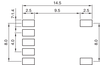
LAND PATTERNS (mm) 推奨ランド寸法
