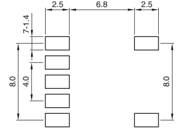
LAND PATTERNS (mm) 推奨ランド寸法
