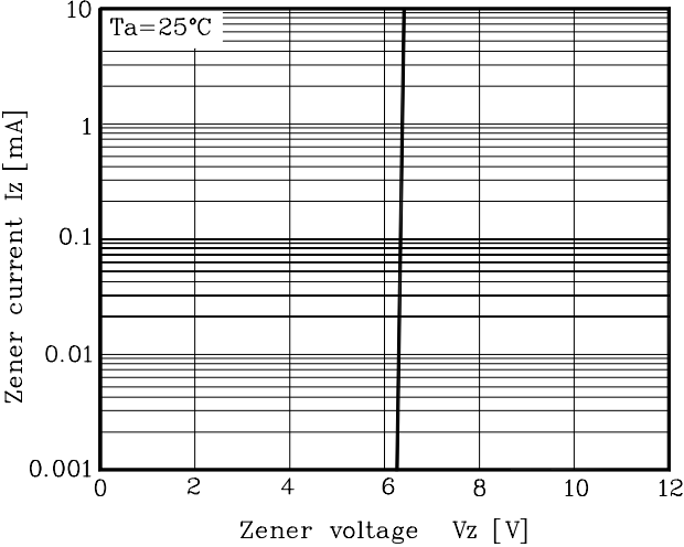
Fig. 2 I_Z - V_Z
