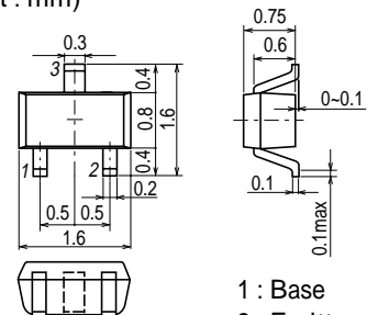
外形図 2106A (unit : mm)
