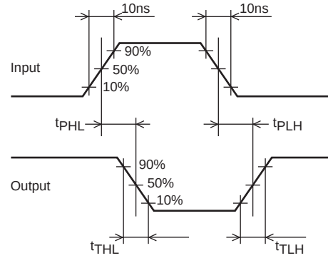
スイッチングタイム波形図
