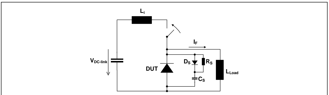
Fig. 7 Test circuit.
