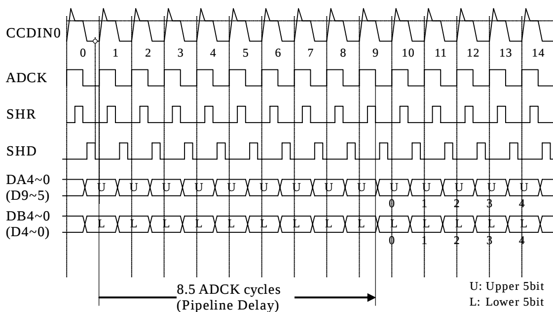
1CH モード時 全体タイミング
