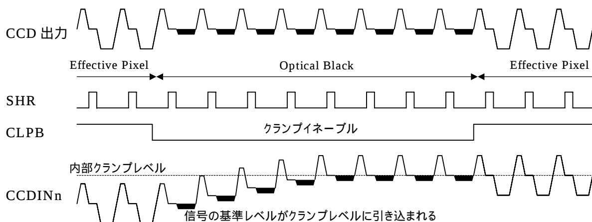
図 8 クランプ動作タイミング概要
