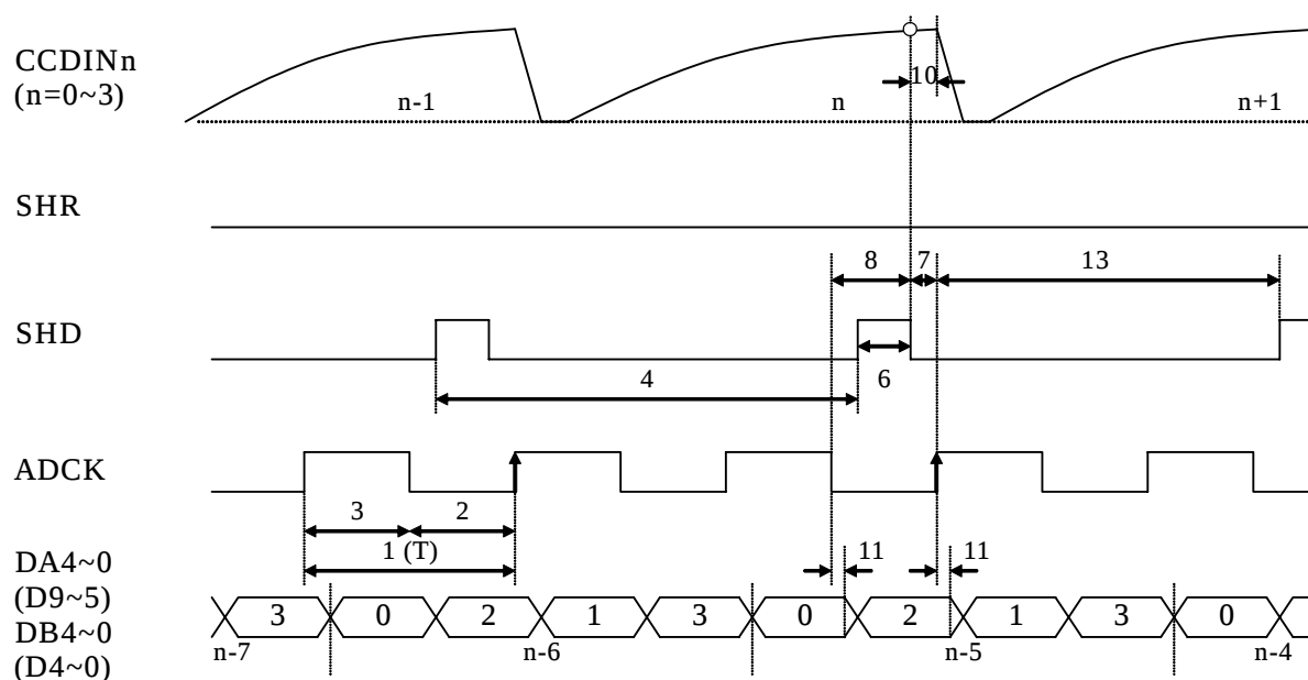
4ch モード時 詳細タイミング
