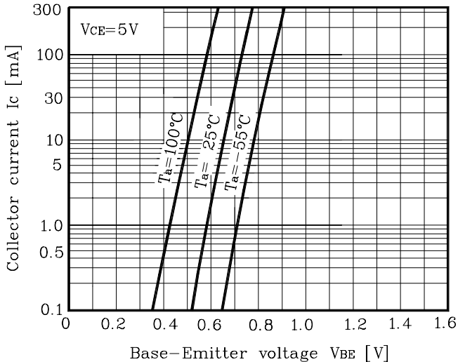
Fig. 2 I_C - V_{BE}
