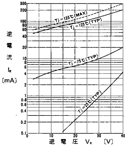
逆特性
