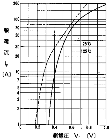
順特性
