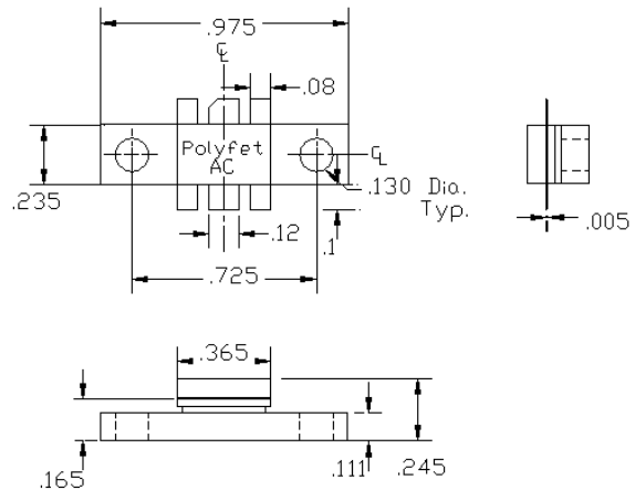
Polyfet AC Package
