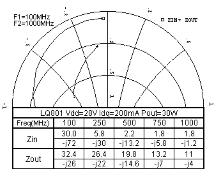
Zin Zout
