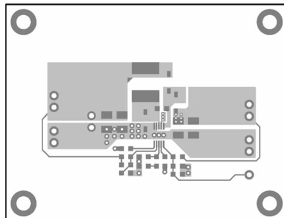
Figure 2—Top Layer
