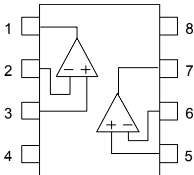
NJM2746M NJM2746V NJM2746RB1 (Top View)
