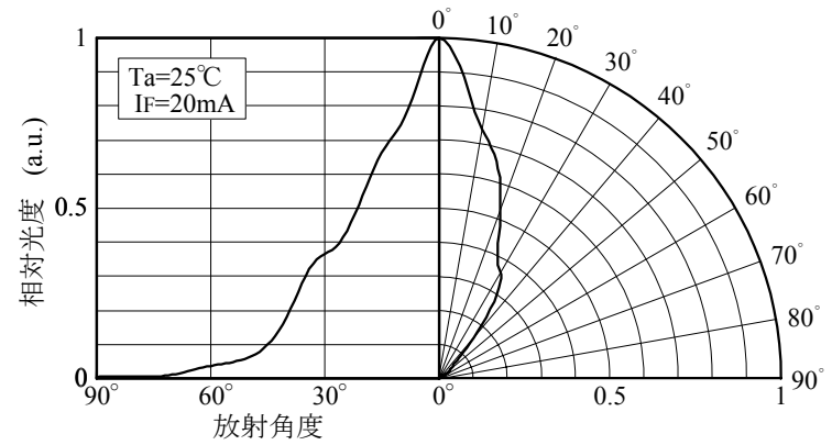
■ 指向特性 (NSPG520S)
