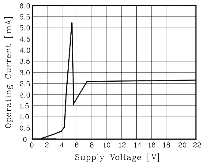
Fig. 2 V_{CC} - I_{CC}
