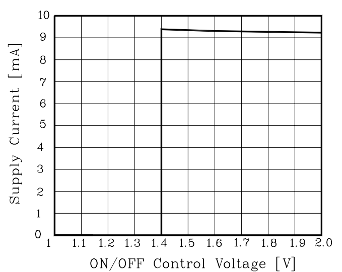
Fig. 8 V_{ENA} - I_{CC}
