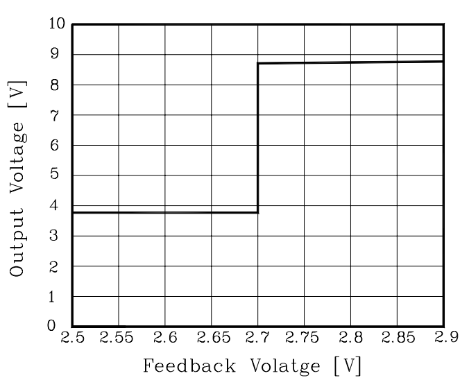
Fig. 7 V_{SCP} - V_{OUT}
