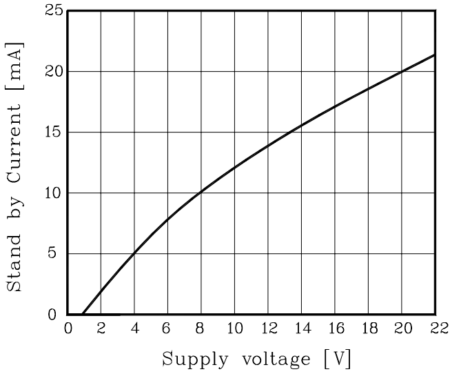
Fig. 1 V_{CC} - I_{SB}
