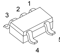
SOT-25
