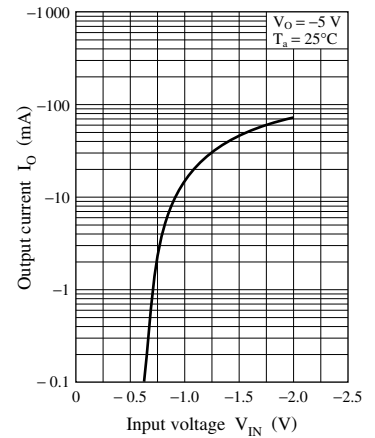
I_O - V_{IN}
