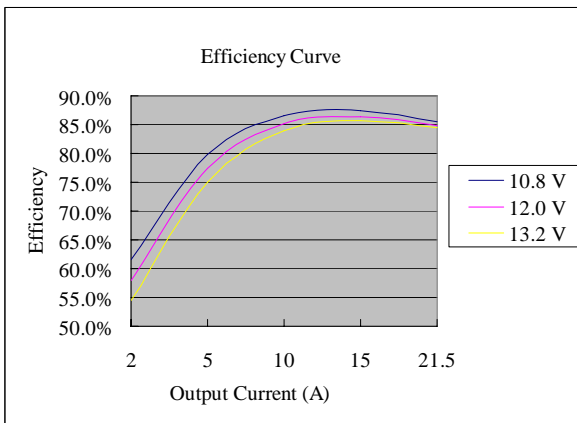
V_o=1.8\text{ V}
