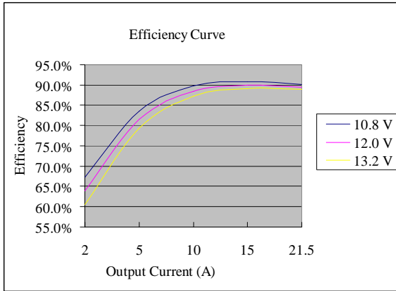
V_o=3.3\text{ V}
