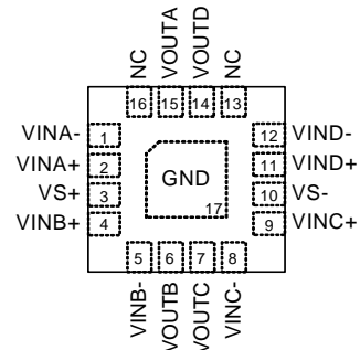
VQFN-16L 4x4
