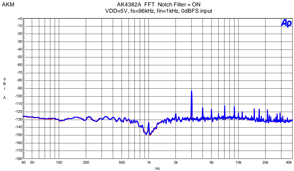
Figure 19. FFT(fin=1kHz, 0dBFS input, Notch)
