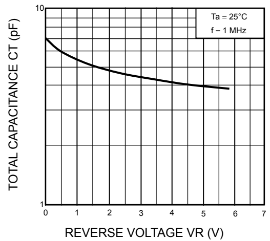
C_T - V_R
