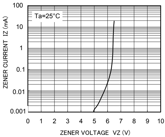
I_Z - V_Z
