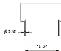
FYD-5021Hx
