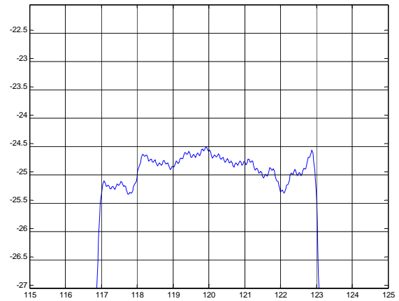
Phase Linearity( f_0 \pm 2.9\text{MHz} )
