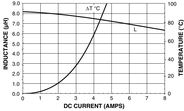
IHLP-2525BD-01 8.2 \mu H
