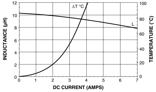
IHLP-2525BD-01 10 \mu H
