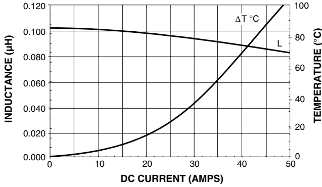
IHLP-2525BD-01 0.1 \mu\text{H}
