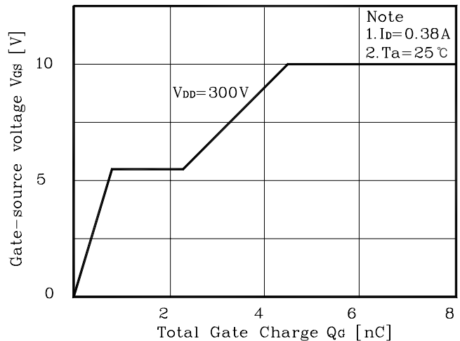
Fig. 6 V_{GS} - Q_G
