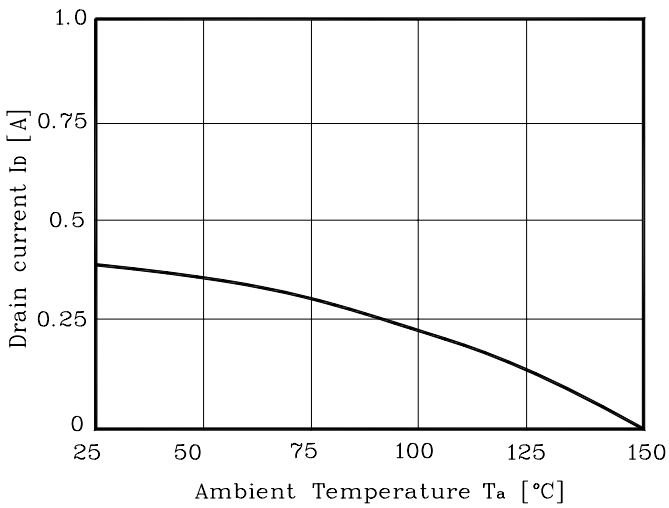
Fig. 9 I_D - T_a
