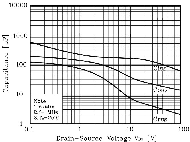
Fig. 5 Capacitance - V_{DS}
