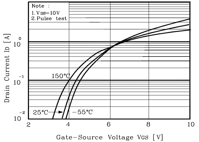
Fig. 2 I_D - V_{GS}
