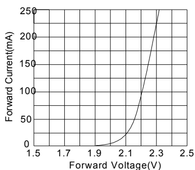
Fig.1 正向电流 Vs. 正向电压
