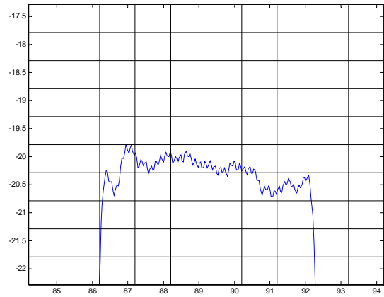
Phase Linearity( f_0 \pm 2.8\text{MHz} )
