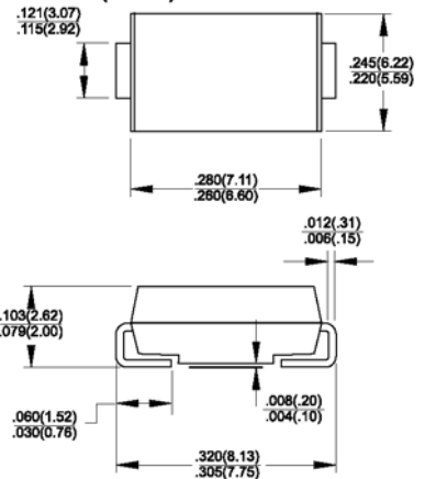
DO-214AB (SMC)
