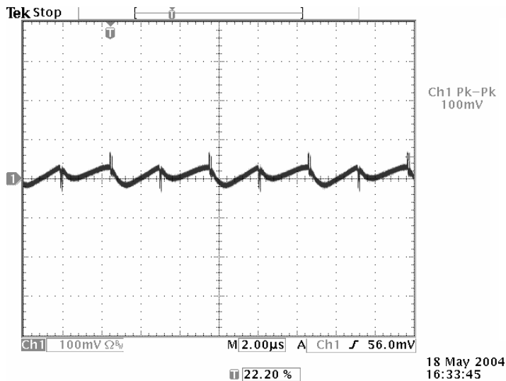
Output Ripple/Noise
