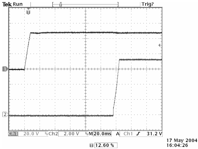
Turn-on from Vin (Enable On)
