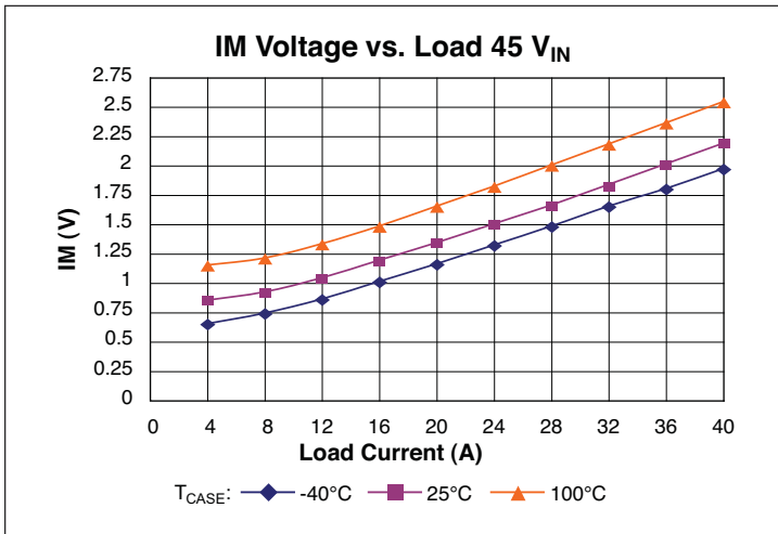
Figure 7 – IM voltage vs. load; 45 V_{IN}
