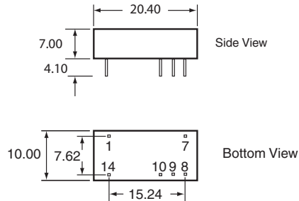
CTDD2010DF-DU3K-1 Footprint
