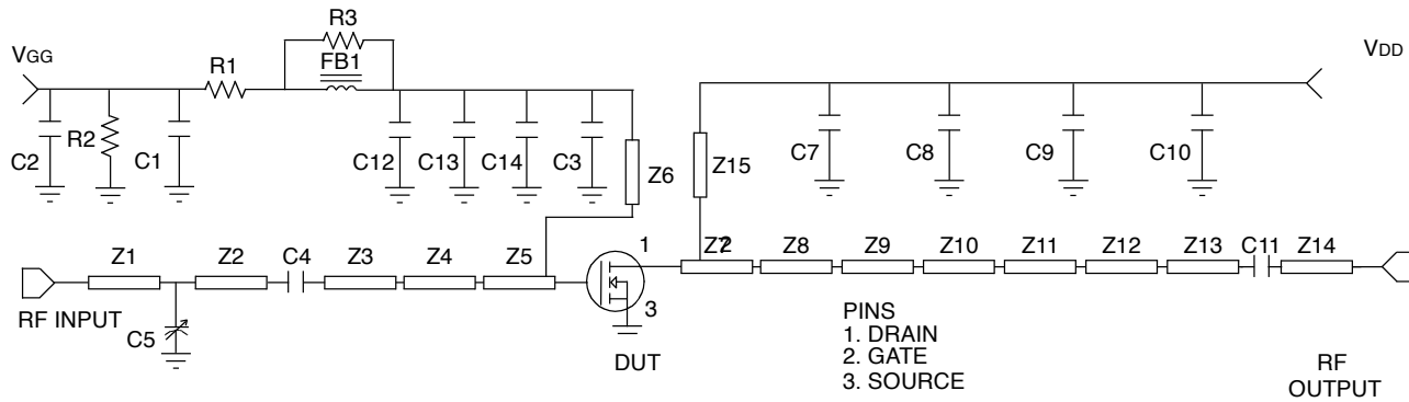
A. Schematic
