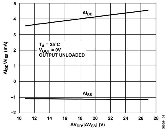
Figure 8. I_{1DD}/I_{1SS} vs. AV_{1DD}/AV_{1SS}
