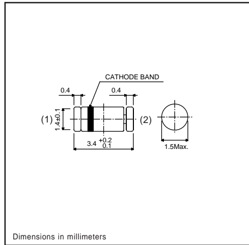
Mini-Melf
