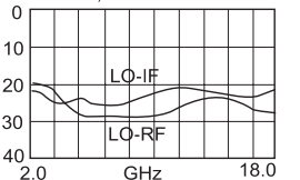
LO to RF, LO to IF Isolation-dB
