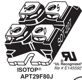
Single die FREDFET
