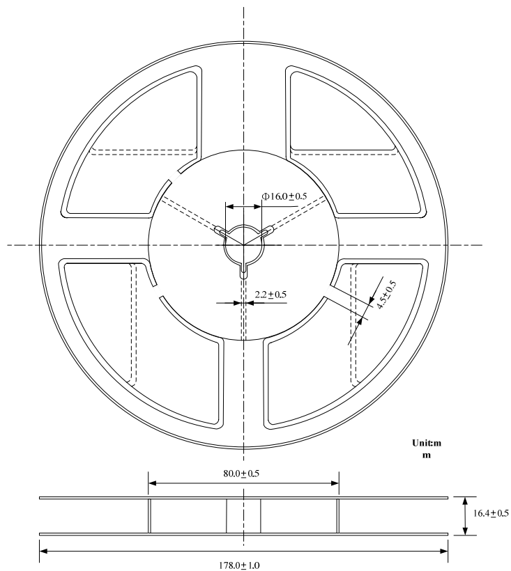
Reel Dimensions
