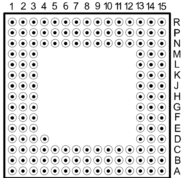
144-Pin CPGA
