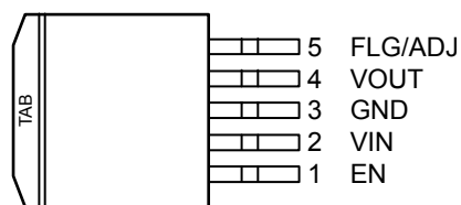
S-PAK-5 (R)
