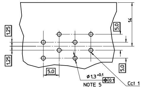
P.C.B. POLARISATION OPTION 'A'
