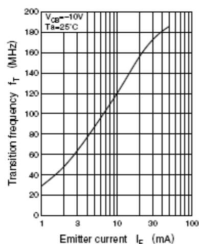
f_T - I_E
