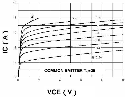
IC - VCE
