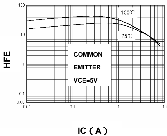
HFE - IC
