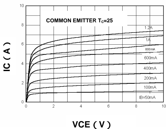
IC - VCE
