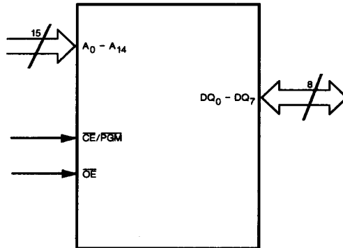
Am27256
