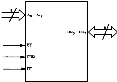
Am2764A
