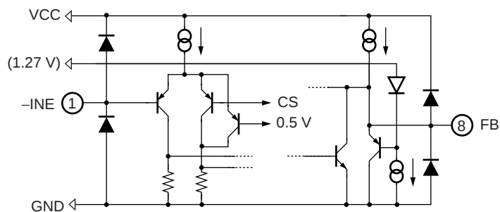
《Error amplifier block》
