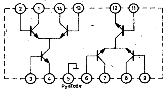
Schemat wewnętrzny /UL 1102/
